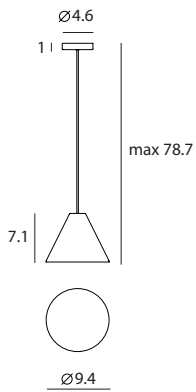
Castle Pendant Cone SQ-185CP E26 1 x Max 77W Gray textile wire Materials : concrete, aluminum Color : concrete Canopy : chrome
