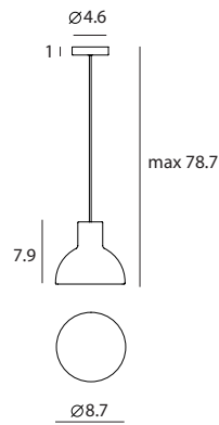
Castle Pendant Bell SQ-3164CP E26 1 x Max 77W Ribbed reflector Gray textile wire Materials : concrete, aluminum Color : concrete Canopy : chrome
