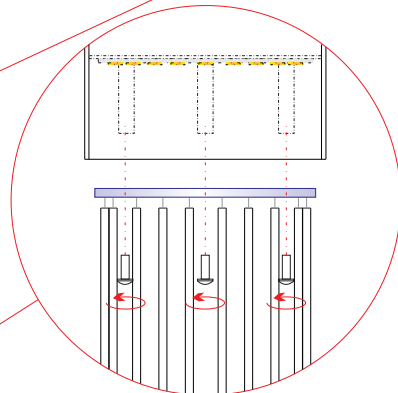
Fissaggio diffusore aste in metallo Diffuser with metal rods fixing
