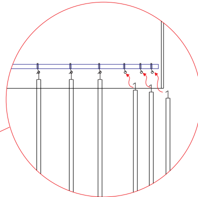
Fissaggio aste in vetro Glass rods fixing
